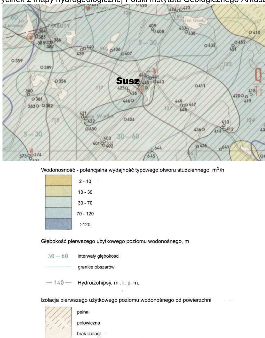
Rysunek 2. Wycinek z mapy hydrogeologicznej Polski Instytutu Geologicznego Arkusz nr 18 - Iława
