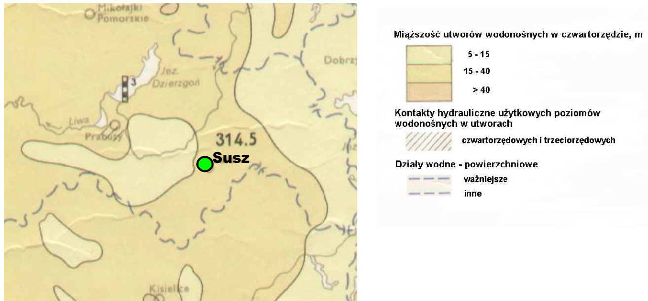
Rysunek 3. Wycinek z mapy hydrogeologicznej Polski Instytutu Geologicznego Arkusz nr 18 - Iława
