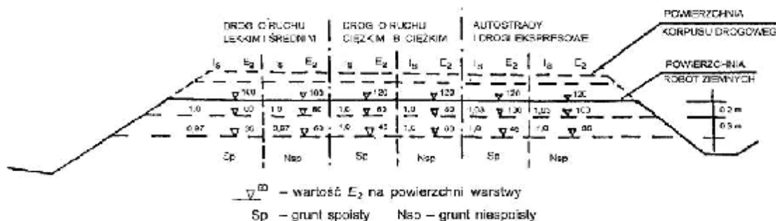
Rysunek 4 – Wartości wymagane w podłożu wykopów: wskaźnika zagęszczenia I_z i wtórnego modułu odkształcenia E_z , megapaskali
