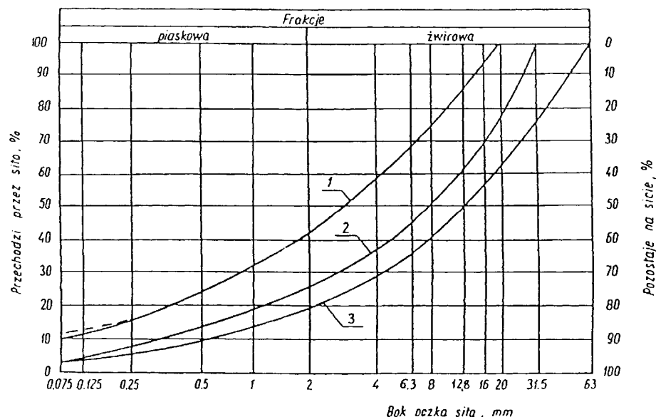
Rysunek 1. Pole dobrego uziarnienia mieszanki przeznaczonych na podbudowy wykonywane metodą stabilizacji
