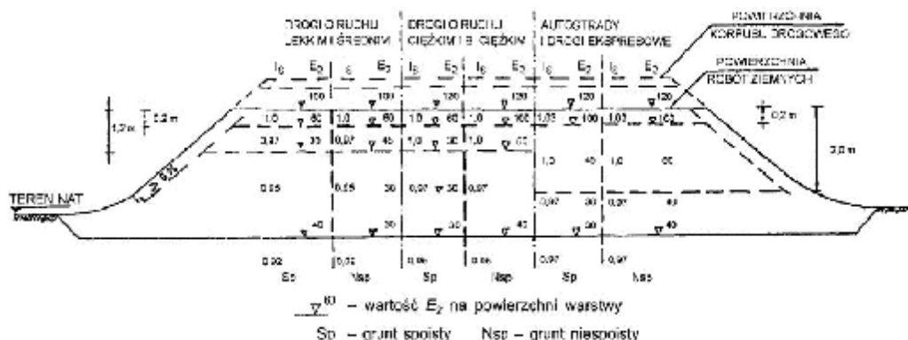
Rysunek 3 – Wartości wymagane w nasypach: wskaznika zagęszczenia I , i wtórnego modułu odkształcenia E_s , megapaskal
