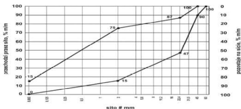
Rys. nr 1 Mieszanka kruszyw 0/31,5 do warstwy podłoża ulepszonego
